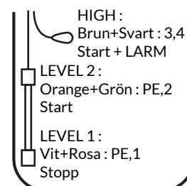
F. NivåPRO ESPS-100 + 1 nivåvippa
