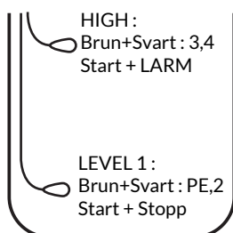
A. 2 nivåvippor
