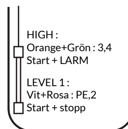
C. NivåPRO ESPS-100
